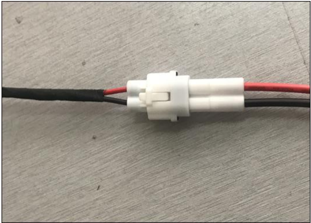
电机接线方法：首先把端头盖线束两边端头颜色一一对应，然后把另一个端头的电机线红色线接红色线，黑色线接黑色线
