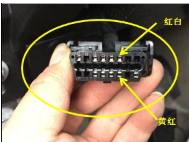
接原车 OBD 接头 把主线束上的红白线与 OBD 第 6 脚相连，黄红线与第 14 脚相连（见箭头）
