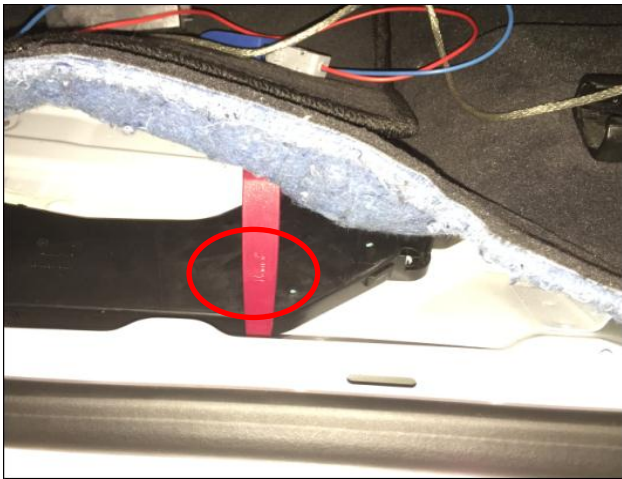
踏板电机穿线孔：掀开此处垫脚海绵、黑色塑料件，看到穿线孔，电机线由车底穿进（圆圈）；左右两边踏板电机穿线孔方法一致；
