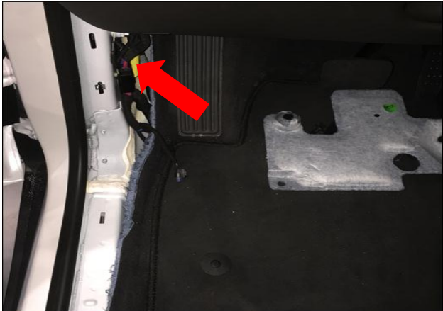
拆内饰件 拆下驾驶室左下脚内饰件（箭头），并妥善保管，后续还原安装。
